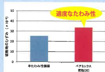
破断時のひずみ (-10°C)
