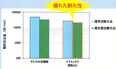
ホイールトラッキング試験結果
