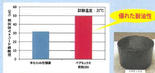
油浸後のマーシャル安定度試験結果
